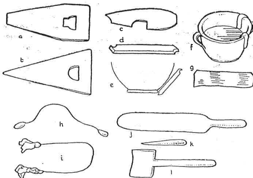
Korongolásnál használt segédeszközök: a—b) lakések bükkfából, illetve vasból (h: 17 és 18 cm); c—e) lenékszégvágók mázasedényhez és alkalmazásuk; f) vízescserép és g) bőrző (h: 18 cm) az edény ajaka simításához; h—l) rézcérnák hegedő acélhúrból; j) lábaslevegő lapát az újabbforma lábasok leemelése (h: 55 cm); k) vágó, lapos felével fedőt s más apró tárgyat vágnak le a korongról, hegyes felével szűrőt lyukasztatnak; l) lapocka az agyag letakarítására (a—b, f—l és l. Madaras, c—d, j—k. Dánfalva)
