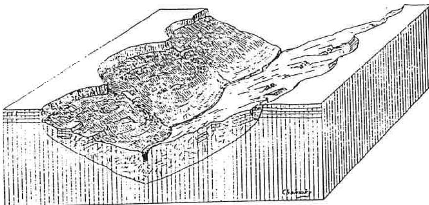
A kajántói völgy tömbszelvénye. Kolozsvártól északra van ez a sűrűdásokkal folyton mozgó völgy.
