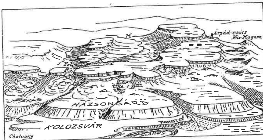
Kolozsvár környékének földfelszíni formái. S = fiatal suvadások ; B = Bercsényi-turistaház ; M = Malomvölgy.
