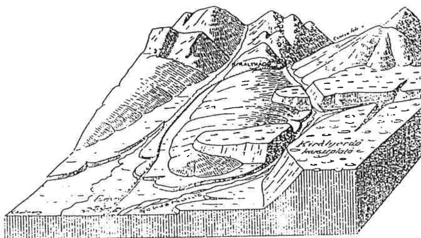
A Királyhágó vázlatos tömbszelvénye.
