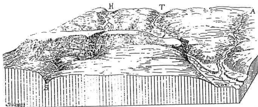
A Torda-hasadék és a Túr-hasadék vázlatos szelvénye. H = Hesdát-patak : T = Túr-patak : A = normális völgy a medencében : S = Sinfalva : Tor. = Torda.
