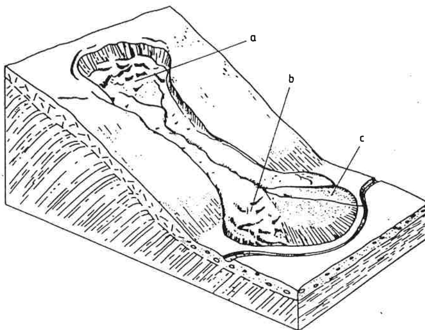
Köpenycsuszamlás (Zaruba-Menci - 1969 - alapján). a = az alapkőzetig kiürült csuszamlásfészek, b = a lecsúszott anyag halmaza, c = a csuszamláshalmaz egy részén a patok hordalékkúpot formált
