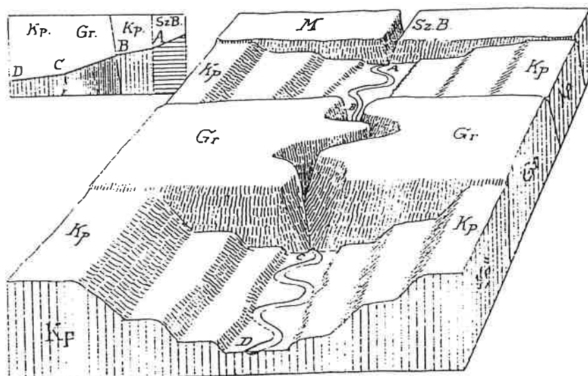
A Meleg-Szamos völgye a Gyalui-havasokou át. M = A Bihar-hegység mészkő-planinája; SzB = Szamosbazár; Kp = laza kristályos palák; Gr = gránit, A, B, C, D = a folyó ki- és belépő pontjai, a baloldali hosszlevény megfelelő pontjainak értelmezésére.
