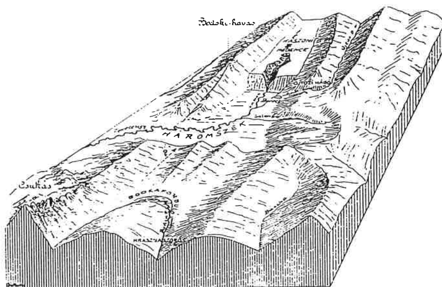
A Háromszéki-medence, a Bodza forduló és a Kászon-medence többszélvénye.
