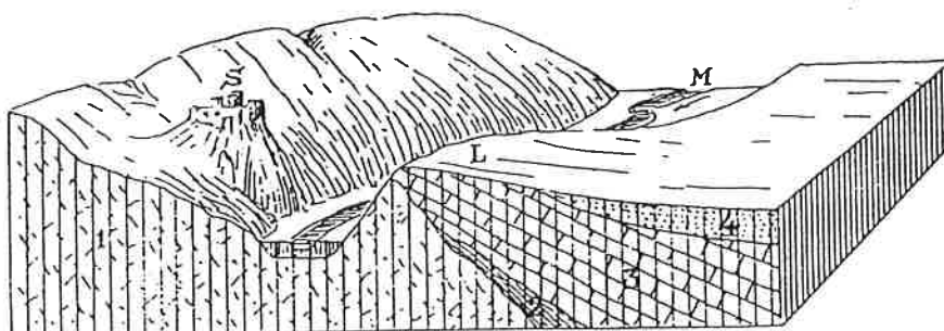
A Maros epigenetikus szurdoka, Sólymos vára és Lippa-vára közt. M = Maros; S = Sólymos vára; L = Lippai-hegy és elpusztult vár; 1. gránit, gnejsz; 2. illit; 3. mészkő; 4. pleisztocénkori agyagok stb. (Id. Lóczy Lajos szelvénye alapján.)
