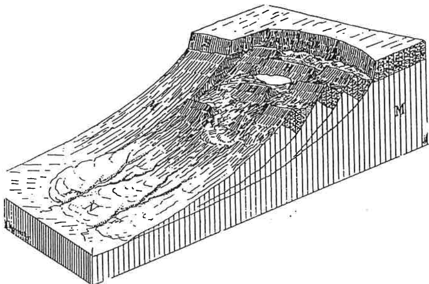
A suvadások általános alakzata. M = mezősegi agyag ; S = szármáciai homokkő ; Sz = a suvadás szakadása ; H, H = hupák, köztük csillog a hepe-tó ; N = a suvadás földfolyása ; F = fiatalon képződött vízmosások.
