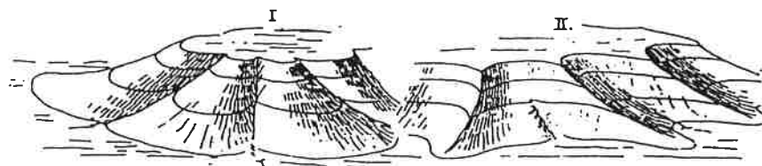
Normális hegylejtő (I.) és suvadásos hegylejtő (II.) vázlatos, szintvonalas tömbszelvénye.
