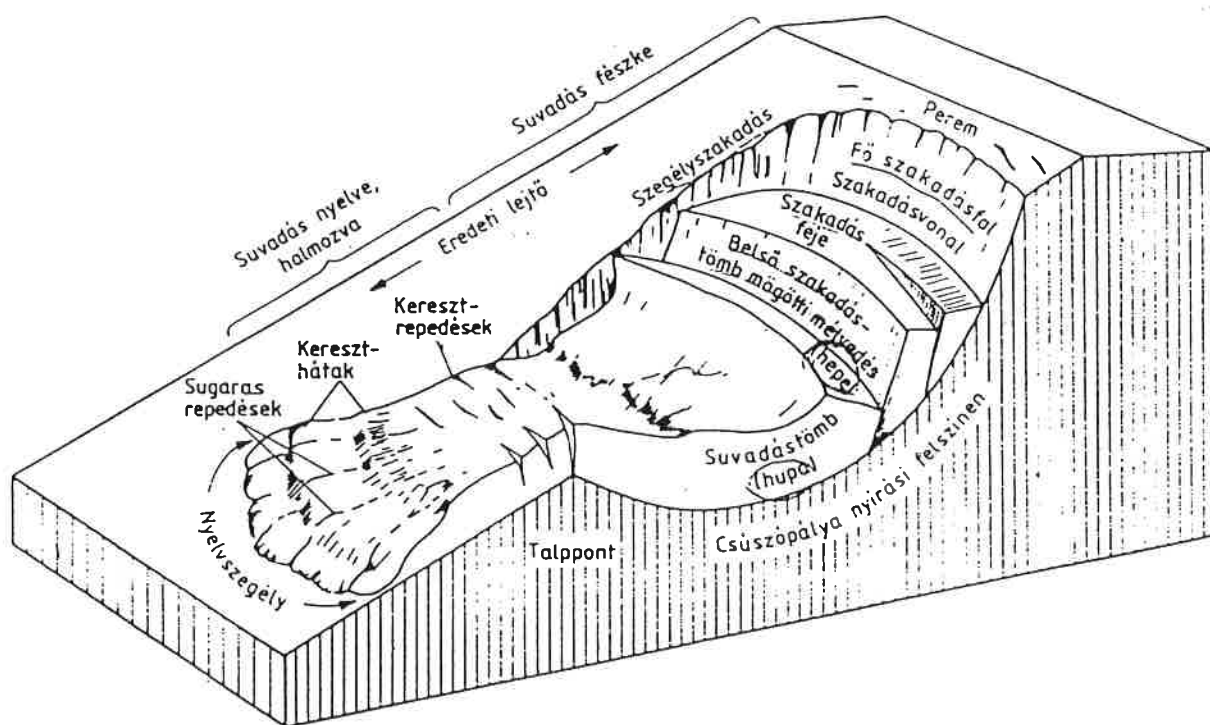
Csuszamlások formai elemei (Varnes, D. J. – 1958 – és Pécsi M. – 1975 – alapján módosításokkal)
