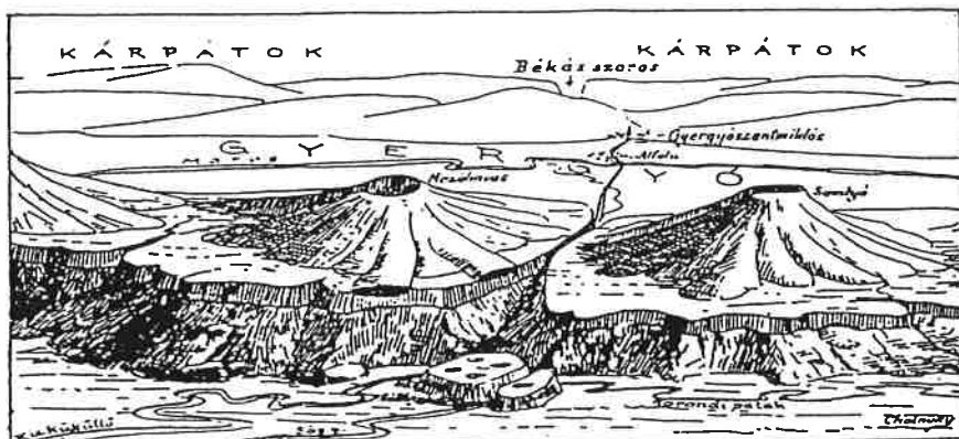
A Hargita-fennsík és a rajta ülő vulkánok vázlatos rajza. Elöl a dolinás parajdi sóhegy, keresztül folyik rajta a korondi Sós-patak; hátul a Gyergyói-medence és a Kárpátok lánc. A szabályos, kúpalakú réteges-vulkánok széles, vulkáni törmelékközzel fedett fennsíkon sorakoznak.
